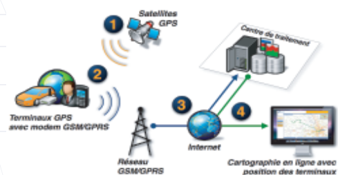
Architecture d'un système de géolocalisation GPS avec remontée des données via le réseau GSM/GPRS
